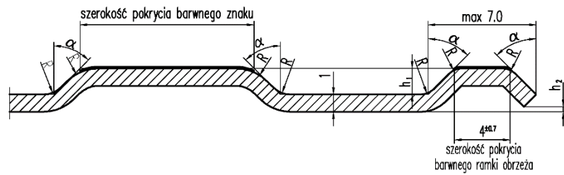
Rysunek 2. Kształt przetłoczeń znaków i ramki obrzeża
